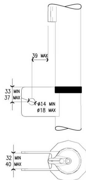
H.1.20 GOOSENECK DIMENSIONS
