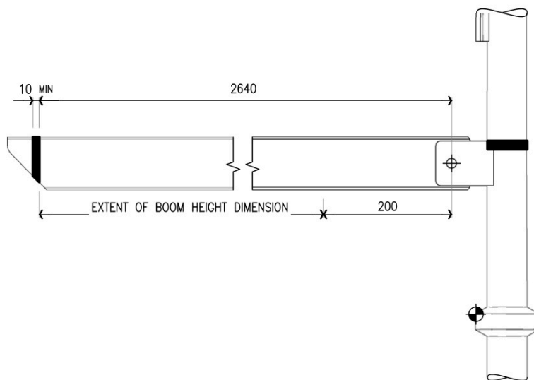
H.1.18 BOOM LAYOUT
